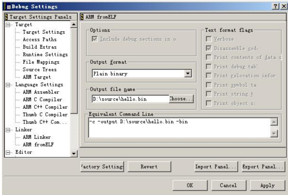
图 11 ARM fromELF 的设置
