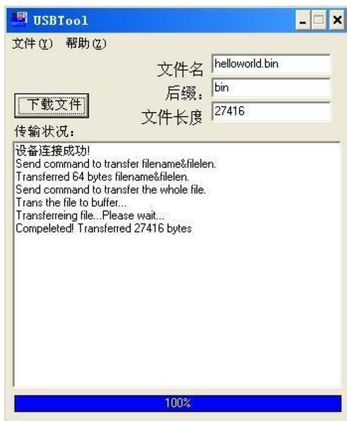
图 27 下载成功界面
