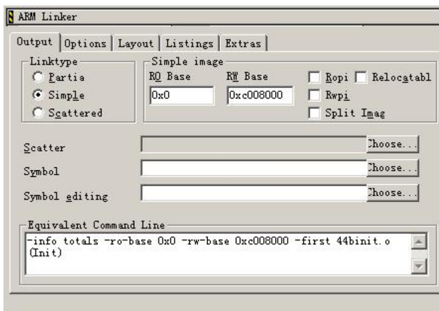
图 28 Entry and Base 设置页
