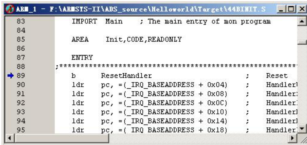
图 21 当前执行代码视窗
