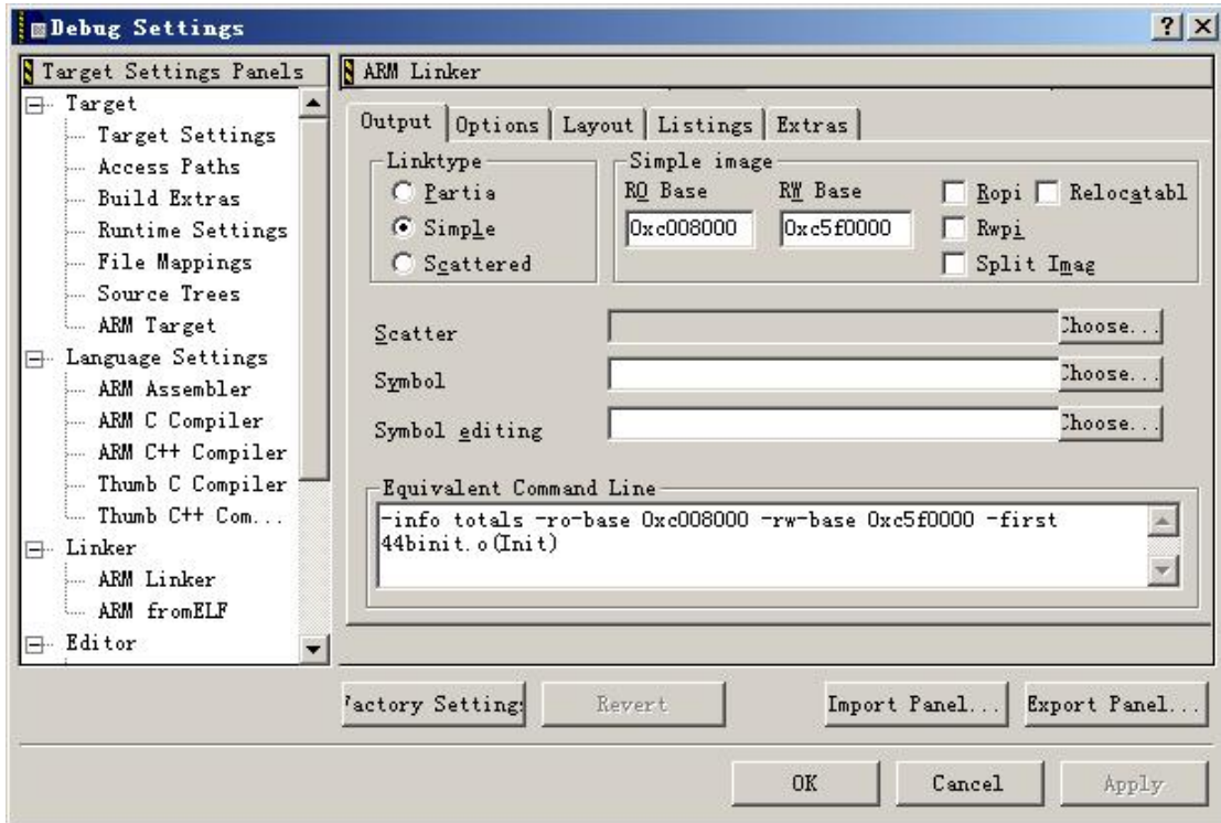
图 10 (a) ARM Linker 的设置
