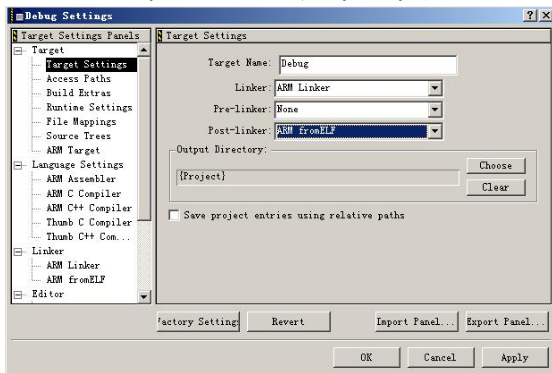
图 9 工程配置对话框——目标设置
