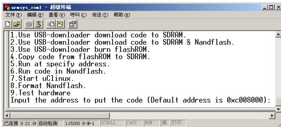
图 27 输入 SDRAM 载入地址
