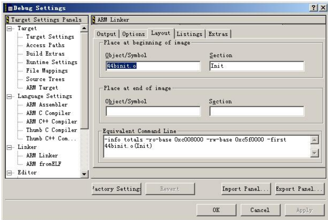
图 10 (b) ARM Linker 的设置
